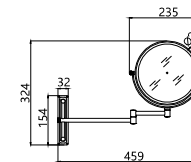
WN860-R
