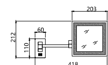
WN812-SL
