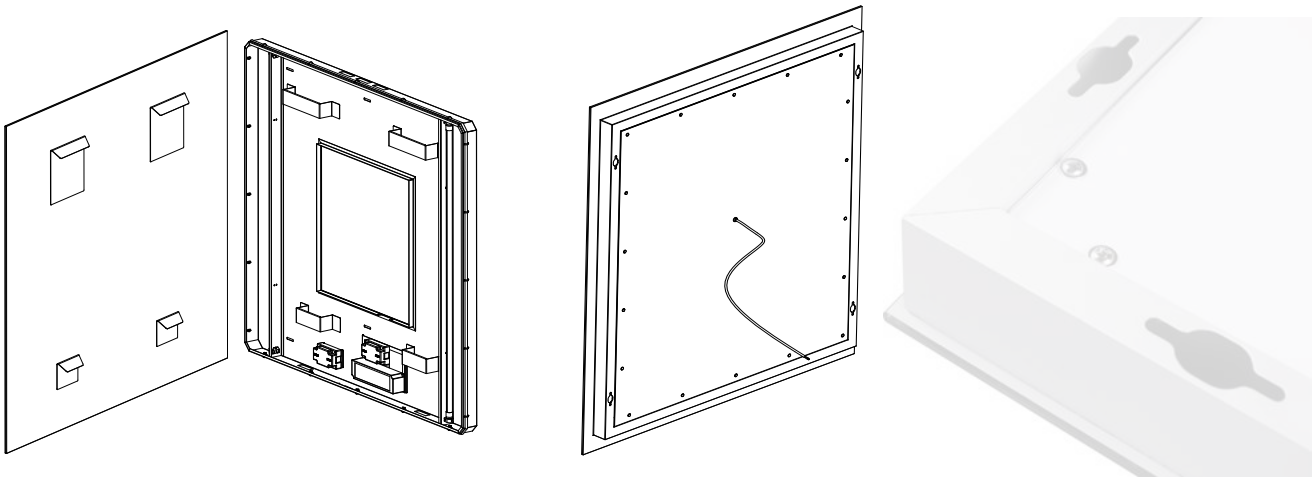
A 分体式（便于安装和维修） A.Split Type (easy to install & maintain) B 整体式（结构可靠，经济性好） B.Integrated Type (economic reliable structure)
